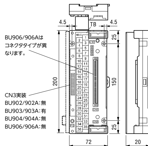
■ TC-net I/O ベース (単位:mm)
