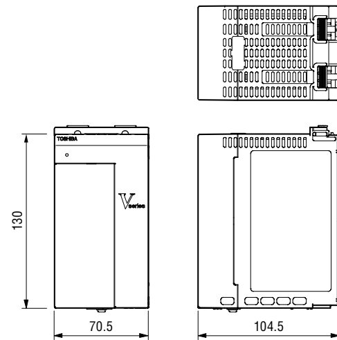
■ 電源モジュール (単位:mm)
