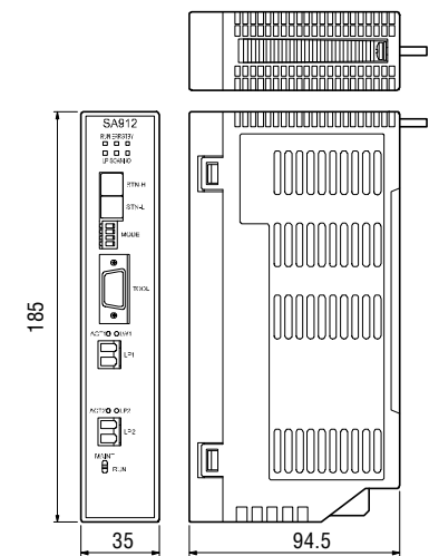
■ TC-net I/O アダプタ (単位:mm)
