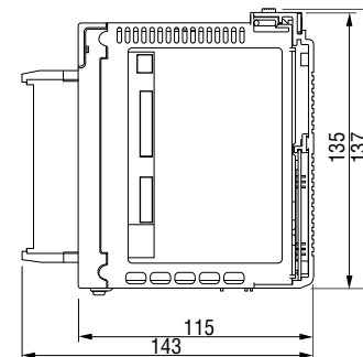
■ G2 I/O モジュール 端子台タイプ (単位:mm)
