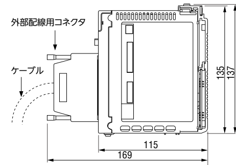
■ G2 I/O モジュール コネクタタイプ (単位:mm)
