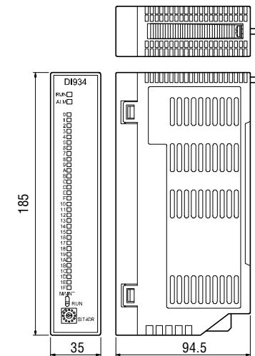
■ TC-net I/O モジュール (単位:mm)
